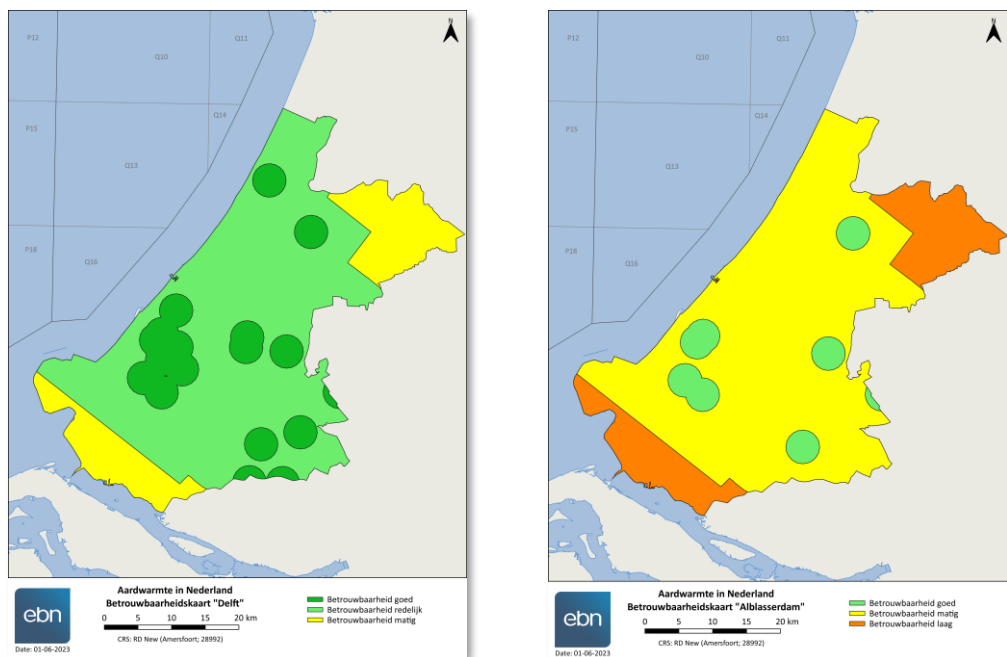
Figuur 3.7: Betrouwbaarheidskaart Delft play (links) en van Alblasserdam play (rechts).
