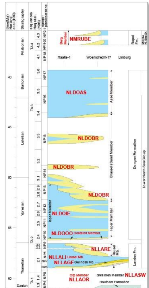
Figuur 7.1: Stratigrafisch overzicht van de Onder-Noordzee Groep. (Bron: Dinoloket; aangepast aan Van Adrichem, Boogaert & Kouwe (1997)).
